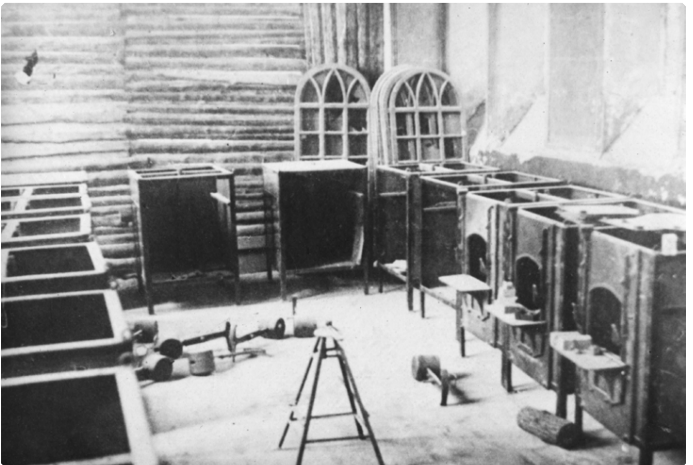
Цех эвакуированного предприятия «Электропечь» в стенах Александро-Невской церкви. 1942 г. БКМ
